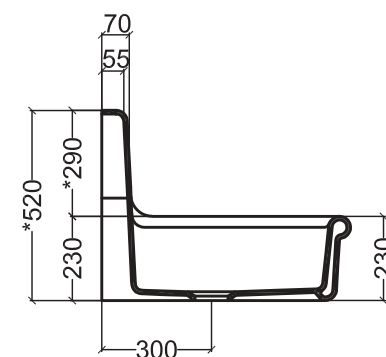
TCK190B/A - cm.90
