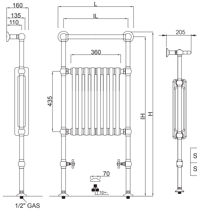
■ SSPVB3 • Radiatore a pavimento con inserto in ghisa mm.1185x545 DT60° Kcal/h 623,6 - Watt 723 Radiateur de sol avec insert en fonte 1185x545mm. DT60° Kcal/h 623,6 - Watt 723 Floor mounted radiator with cast iron insert 1185x545mm. DT60° Kcal/h 623,6 - Watt 723
