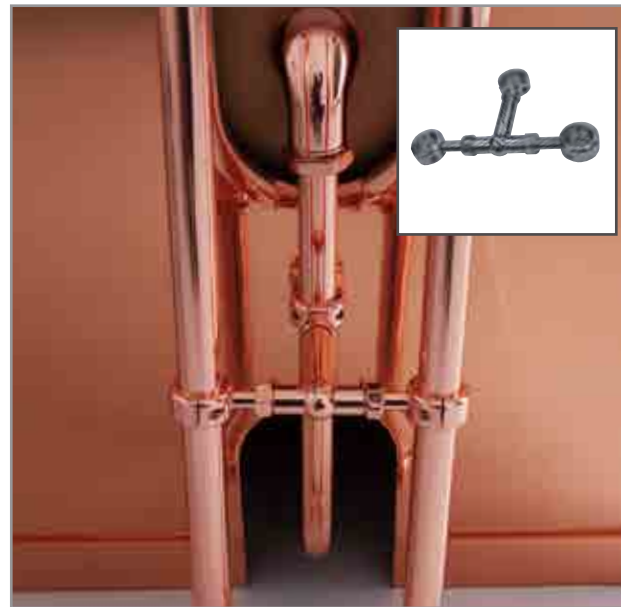
■ STBT • Staffa fissaggio gambe gruppo vasca Fixation colonnes pour RV111/112 Column attachment for RV111/112
