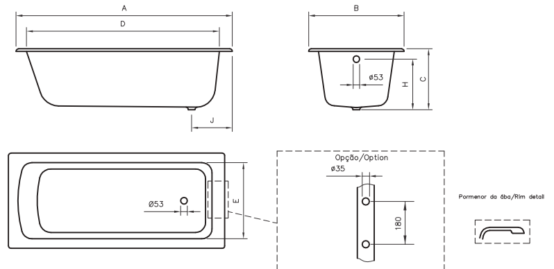
DIMENSIONI - DIMENSIONS (mm)
