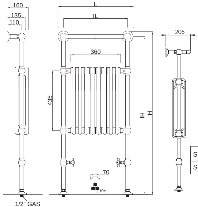
■ SSPVB3CR • Radiatore a pavimento con inserto in ghisa mm.1185x545 DT60° Kcal/h 623,6 - Watt 723 Radiateur de sol avec insert en fonte 1185x545mm. DT60° Kcal/h 623,6 - Watt 723 Floor mounted radiator with cast iron insert 1185x545mm. DT60° Kcal/h 623,6 - Watt 723
