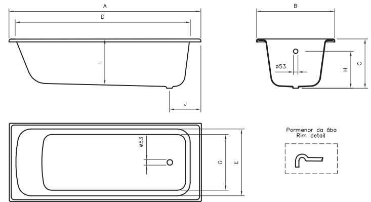
DIMENSIONI - DIMENSIONS (mm)
