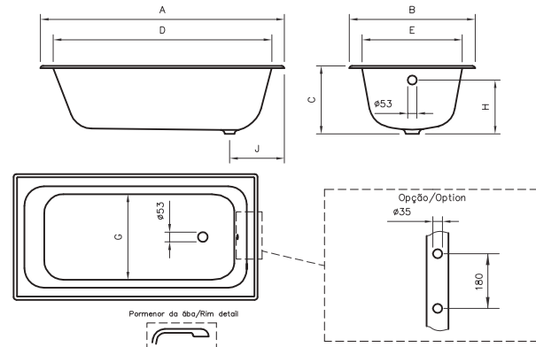
DIMENSIONI - DIMENSIONS (mm)
